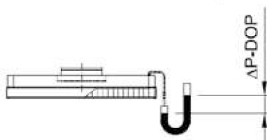
Plenumdan DOP musluklu DOP tap on Plenum
